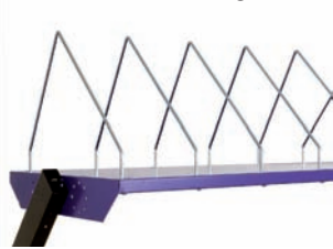
Ablageboden mit 9 Stahlbügeln
