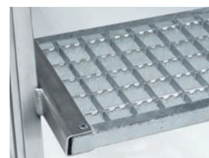
Stufen- und Plattformausführung Stahl-Gitterrost
